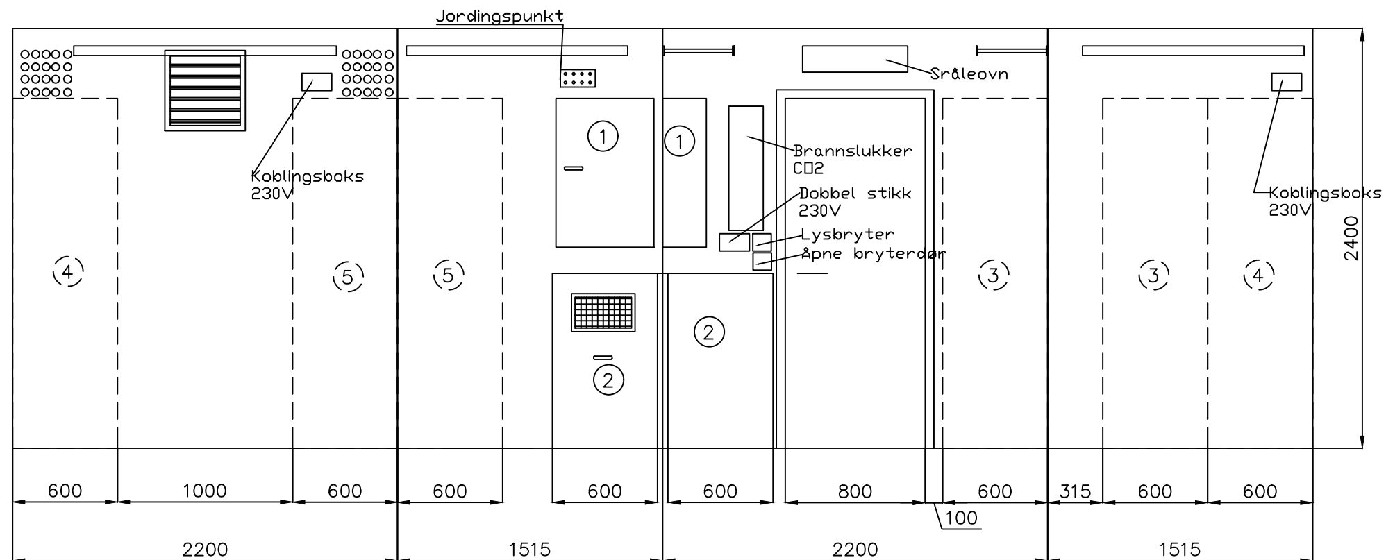
SNITT 1:30
