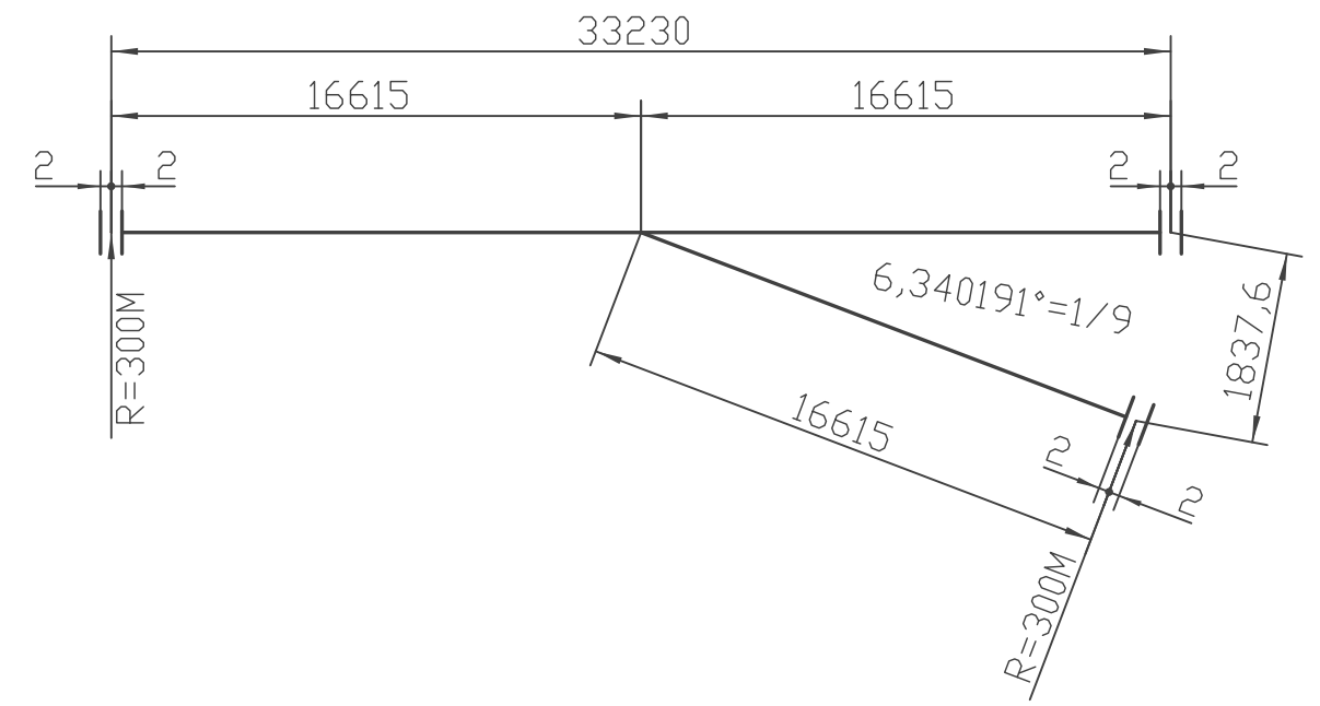
GEOMETRISK SKJEMA
